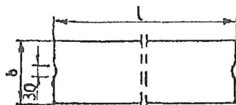
Rys. 1. Wymiarowanie krawężników
