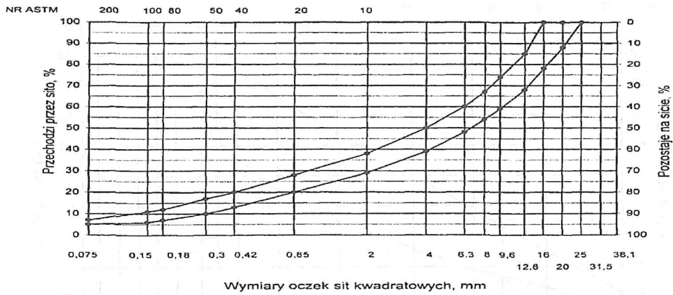
Rys. 4. Krzywe graniczne uziarnienia mieszanki mineralnej BA od 0 do 20 mm do warstwy ścieralnej
